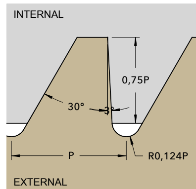
SG DIN 513
