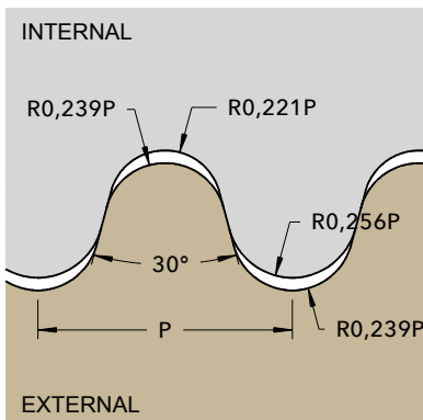
Round DIN 405
