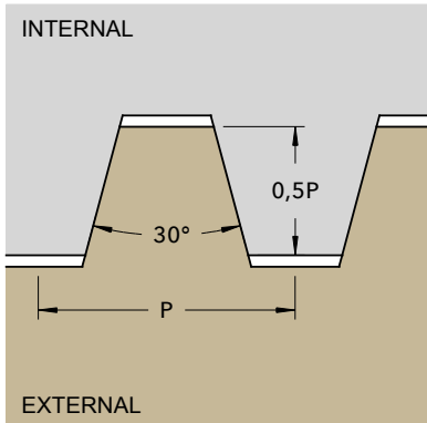
Trapez DIN 103
