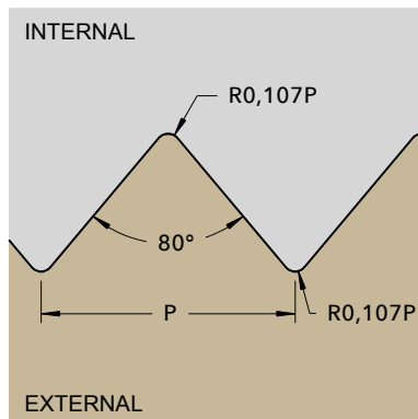
PG DIN 40430
